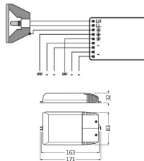
Scheda tecnica Osram PTi 70/220-240 I
